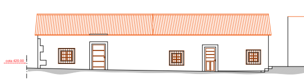
Alçado - OO
