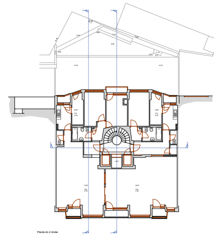
Planta do 2 Andar
