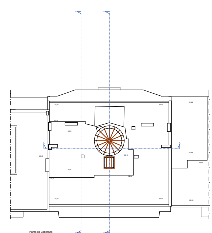
Planta da Cobertura
