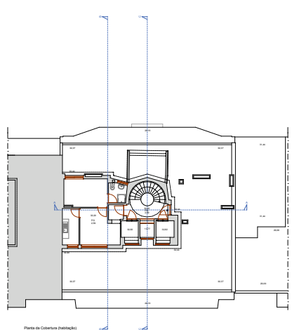
Planta da Cobertura (habitação)
