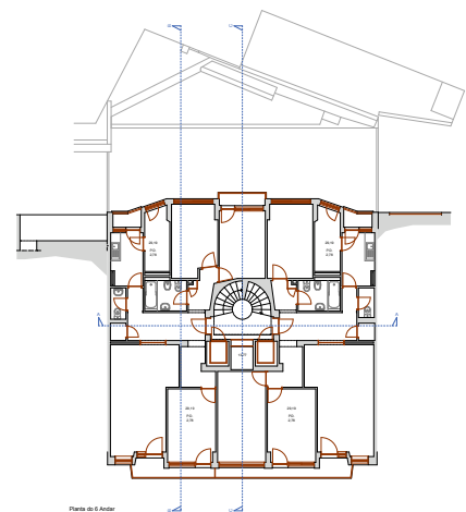
Planta do 6 Andar
