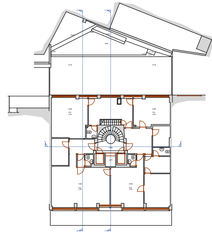
Planta do 1 Andar
