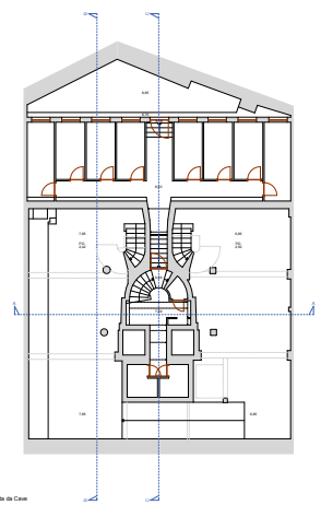
Planta da Cave
