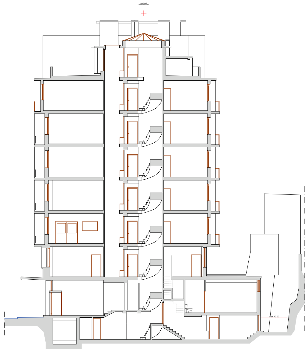
Corte CC
