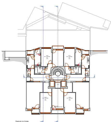
Planta do 4 e 5 Andar
