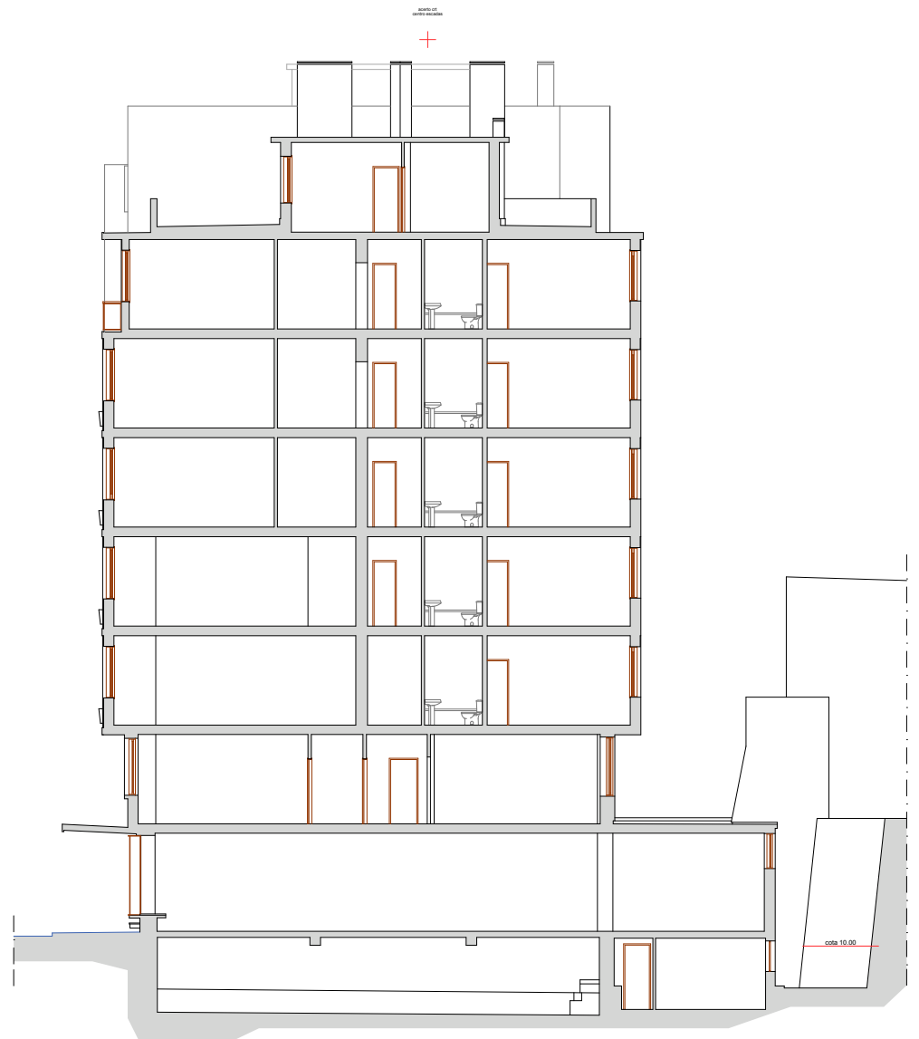
Corte BB
