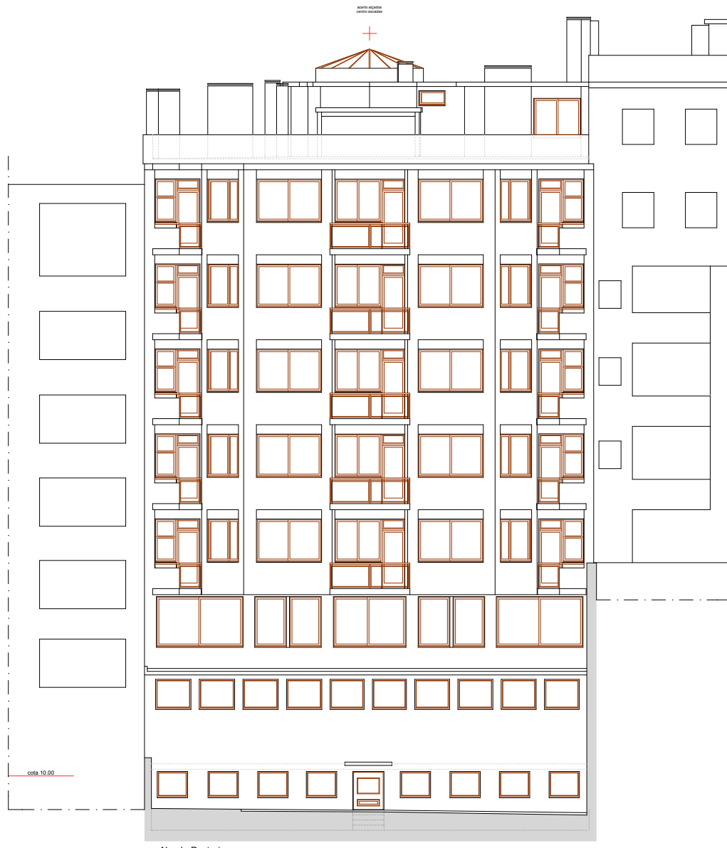
Alçado Posterior
