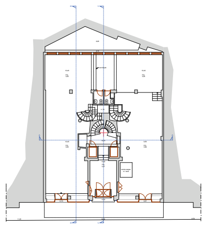
Planta do R/C
