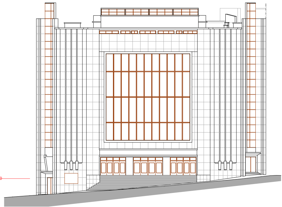
ALÇADO NORTE
